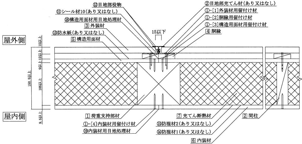
水平断面詳細図 (縦目地仕様 タイプ1)
