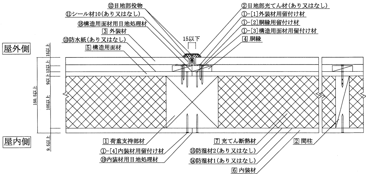
(縦目地仕様 タイプ2)
